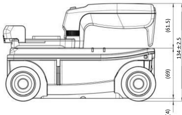
図4 外形図
